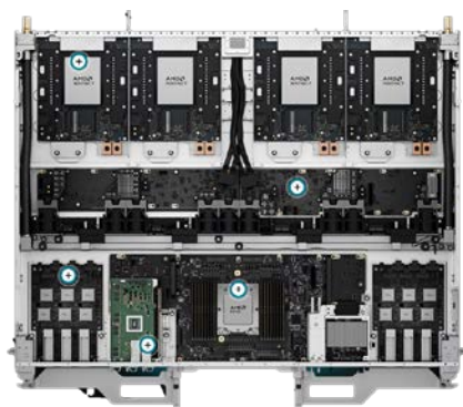
圖 10: AMD 的 Helios 機櫃 (採用 MI450 GPU) 使用水冷系統
