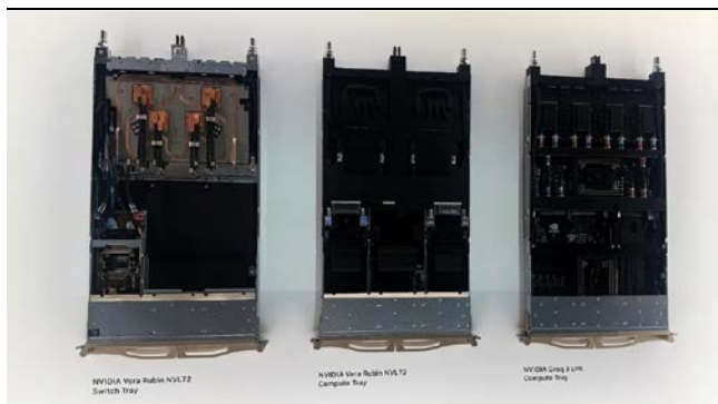
圖 4：Nvidia (美) Vera Rubin 液冷平台
