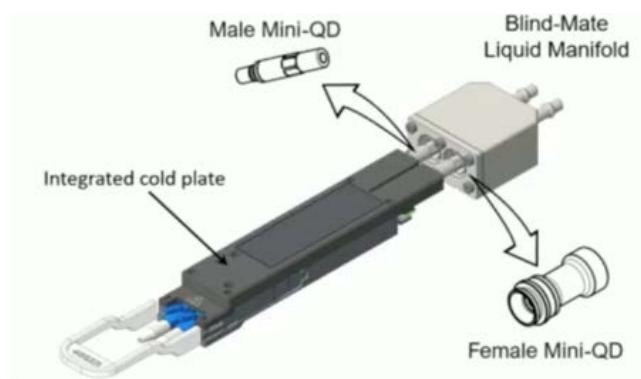
圖 11: 用於 OSFP 的 Mini QD 設計
